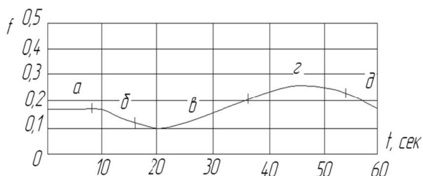
Рис. 1. Залежність сили тертя від часу ковзання по поверхні.
