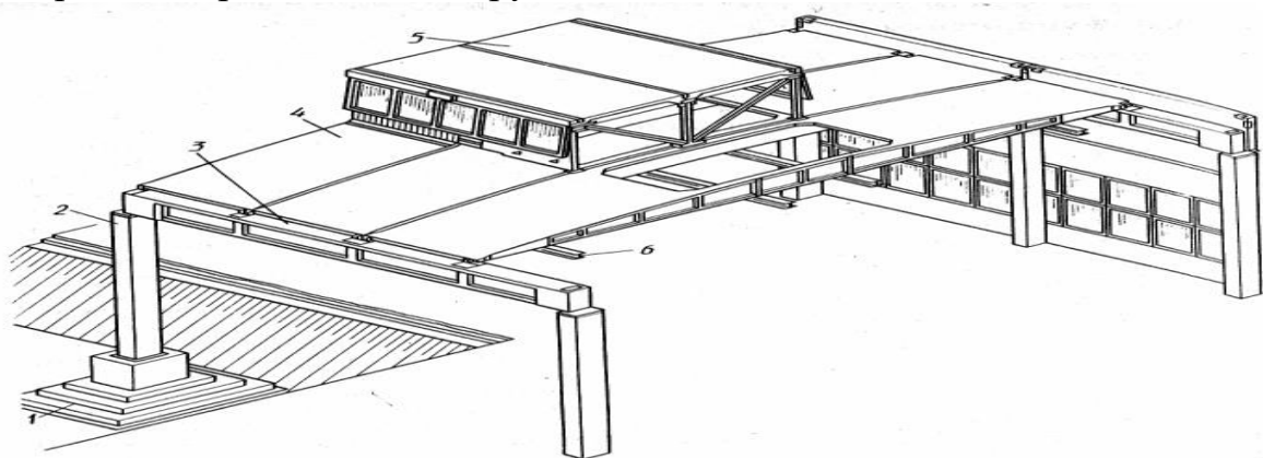
Рис. 5. Залізобетонний каркас з плитами «на проліт».
