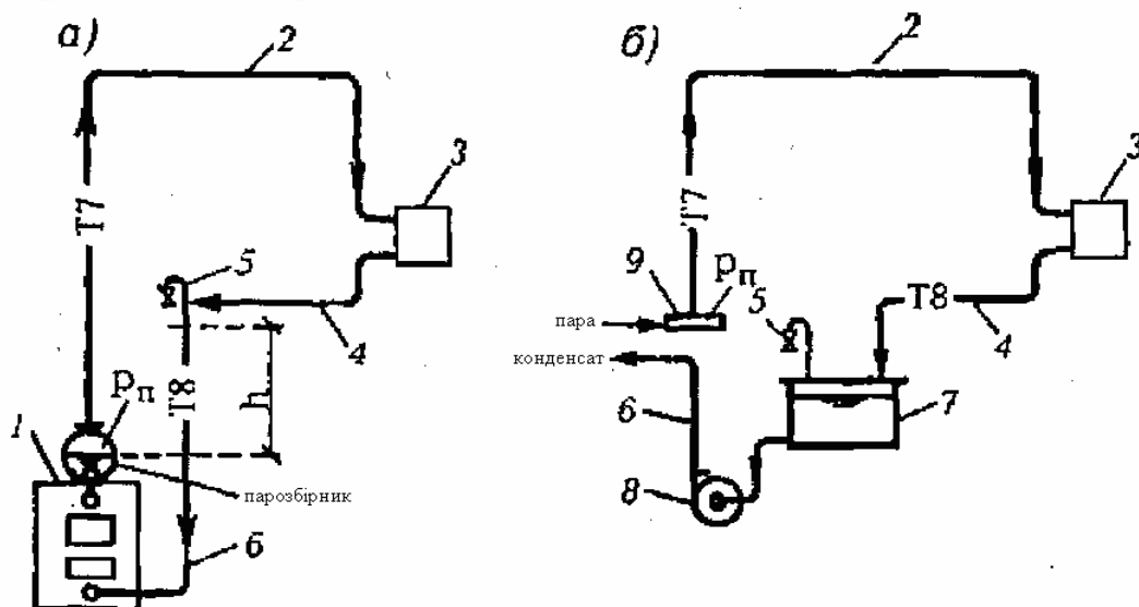
Рис. 14 Схеми системи парового опалення: а – замкнута схема; б – розімкнена схема; 1 – паровий котел з парозбірником; 2 – паропровід (Т7); 3 – опалювальний прилад; 4 і 5 – самопотоковий і напірний конденсатопроводи (Т8); 6 – повітровипускна труба; 7 – конденсатний бак; 8 – конденсатний насос; 9 – паророзподільний колектор.
