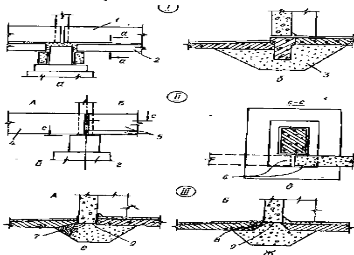
Рис. 9. Варіанти конструкцій панельних стін
