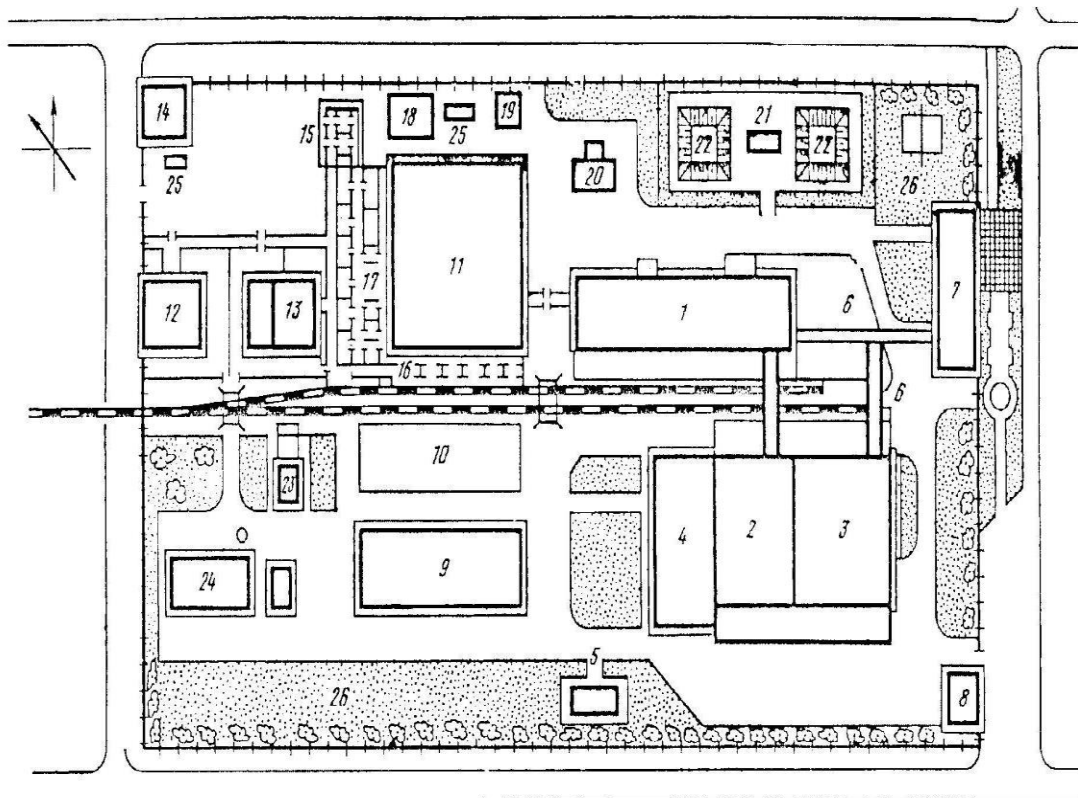
Рис. 2. Генеральний план типового м'ясокомбінату (триповерховий)
